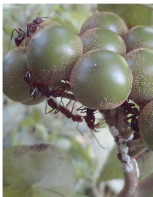
17 Solanum stramonifolium
