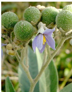
16 Solanum stipulaceum
