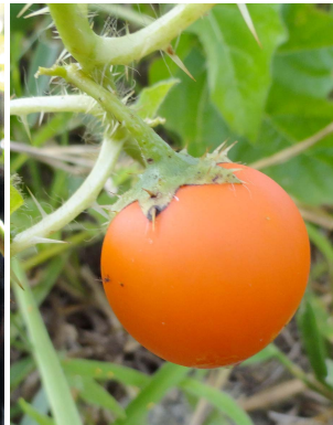
5 Solanum capsicoides
