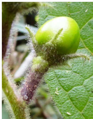
13 Solanum reflexiflorum
